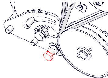
Fig. 27B - Loosen the tie-bar bolt.
