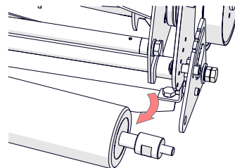
Fig. 27C - Remove the roller.
