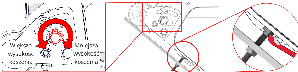
Rys. 8F — Obrócenie koła zębatego, podnosząc jednocześnie drążek regulacyjny. Przerwać, gdy łeb znajdzie się na równi z ostrzem noża lub w jego zasięgu
