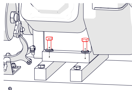
Rys. 17B — Odkręcenie śrub mocujących silnik do wsporników
