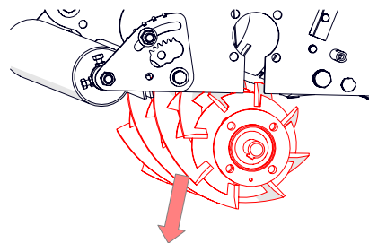
Rys. 18J — Wyjęcie cylindra z maszyny
