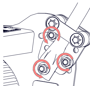
Rys. 10B — Odkręcanie nakrętki wewnętrznej
