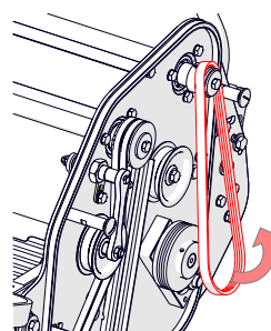
Rys. 16I — Zdjęcie i wymiana paska
