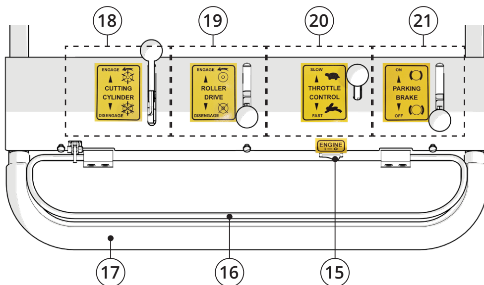
Fig.5. Przegląd elementów sterujących.
