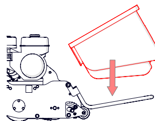
Rys. 2B — Mocowanie kosza na trawę.
