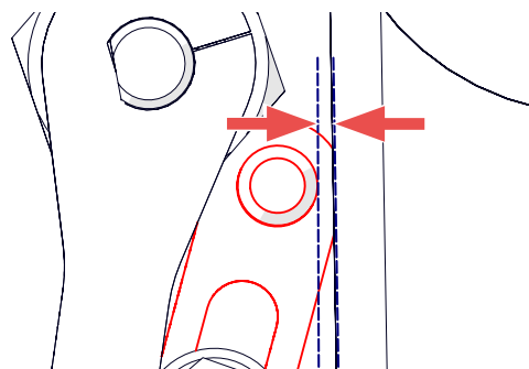
Rys. 24B — Gdy koło pasowe jest załączone, należy zachować bardzo niewielką szczelinę między kołkiem a paskiem
