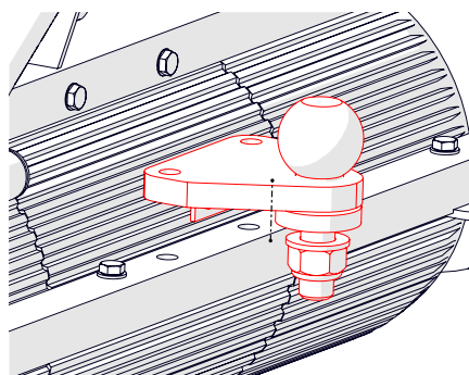
Rys. 28A — Zakładanie wspornika kuli haka holowniczego
