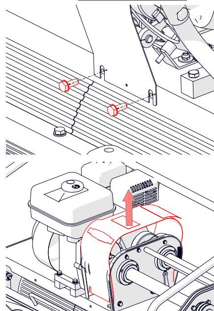
Rys. 17A — Demontaż osłony skrzyni biegów
