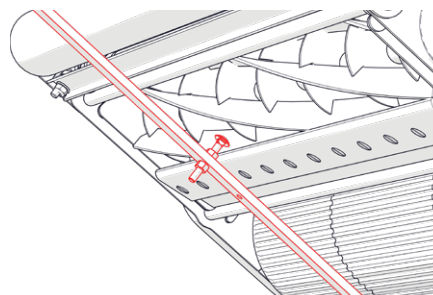
Rys. 8G — Powtórzenie czynności po drugiej stronie
