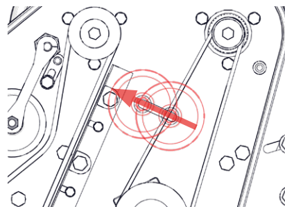
Rys. 16H — Poluzowanie koła napinającego
