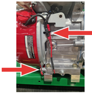
Rys. 17C — Odłączenie przewodów silnika
