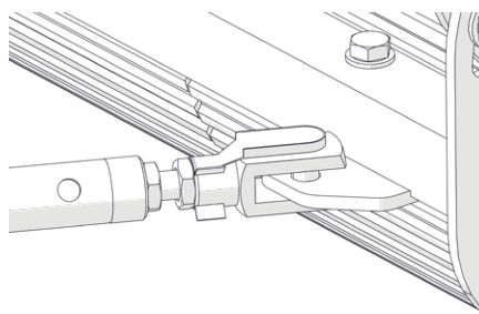
Rys. 28B — Wkładanie śrub od spodu i dokręcanie śrub
