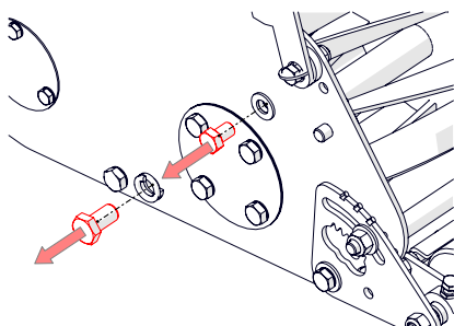
Rys. 18F — Odkręcenie śrub sześciokątnych ostrza tnącego po prawej stronie
