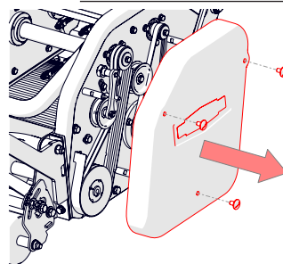
Rys. 18A — Odkręcenie 3 zewnętrznych śrub i zdjęcie pokrywy
