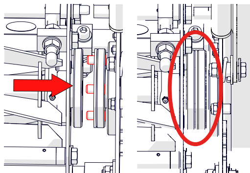
Rys. 7E — Wsuniecie nowej kasety i jej przesunięcie w bok, tak aby zazębiła się z trzema kołkami
