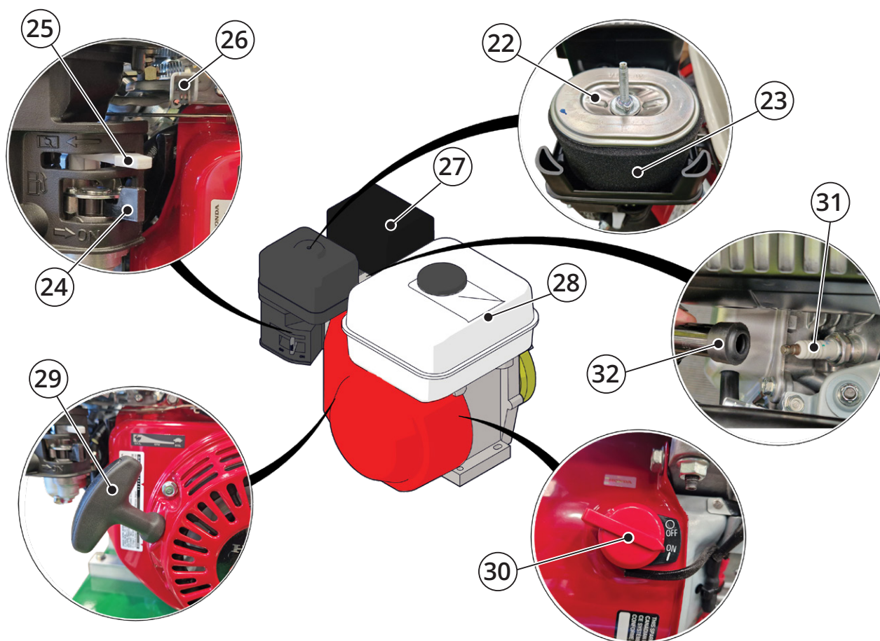
Fig.6. Przegląd elementów silnika.
