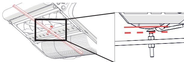
Rys. 8D — Ustawienie drążka regulacyjnego i sprawdzenie odległości między górną krawędzią ostrza tnącego a dolną krawędzią łba śruby. W tym przykładzie łeb śruby znajduje się poniżej ostrza tnącego, co oznacza, że aktualna wysokość koszenia maszyny jest za duża i należy ją zmniejszyć.
