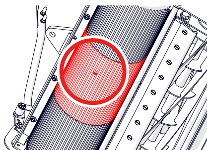
Rys. 23B — Otwór odpływowy wałka skierowany w dół
