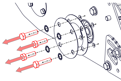
Rys. 18I — Odkręcenie śruby mocującej cylinder po prawej stronie
