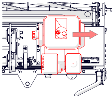
Rys. 17D — Odsunięcie silnika od sprzęgła
