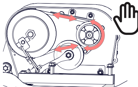
Rys. 17I — Sprawdzanie, czy napięcie jest prawidłowe, poruszając ręcznie kołem pasowym
