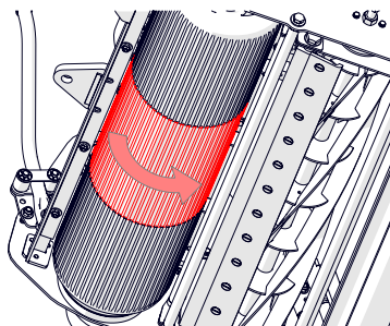
Rys. 23A — Obrócenie wałka środkowego
