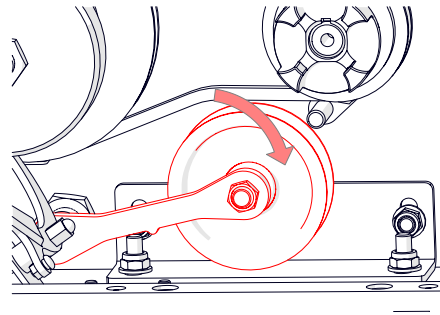
Rys. 17H — Wyregulowanie koła pasowego tak, aby pasek nie stykał się z nim w stanie odłączonym
