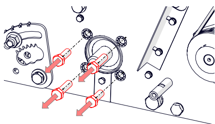
Rys. 18G — Wyjęcie ostrza tnącego z maszyny
