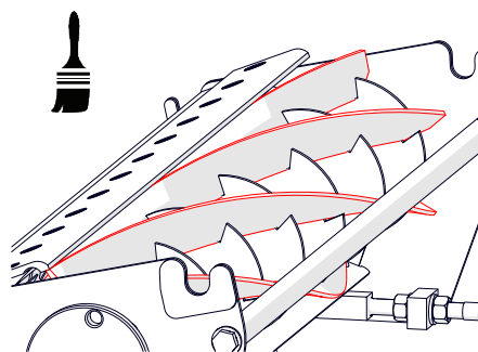
Rys. 19A — Nakładanie pasty na ostrza
