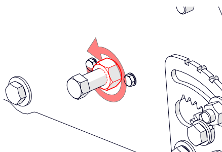
Rys. 7A — Poluzowanie nakrętki zabezpieczającej śruby mocującej
