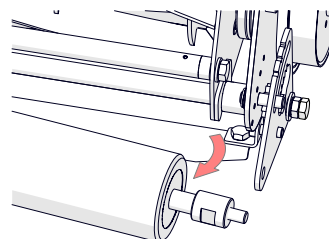
Rys. 27C — Wyjęcie wałka
