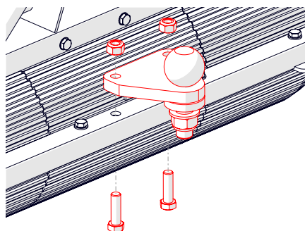
Rys. 28B — Wkładanie śrub od spodu i dokręcanie śrub
