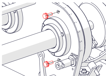
Rys. 17D — Odsunięcie silnika od sprzęgła
