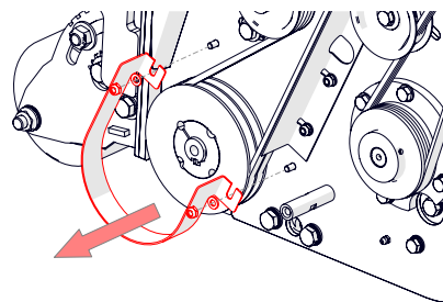
Rys. 18A — Odkręcenie 3 zewnętrznych śrub i zdjęcie pokrywy
