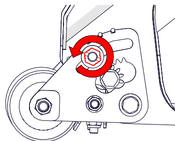
Rys. 8E — Poluzowanie górnej nakrętki zaciskowej krawędzi wałka
