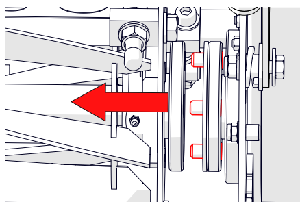
Rys. 7C — Przesunięcie kasety, aż będą widoczne kołki
