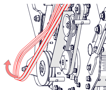
Rys. 18C — Zdjęcie i wymiana paska
