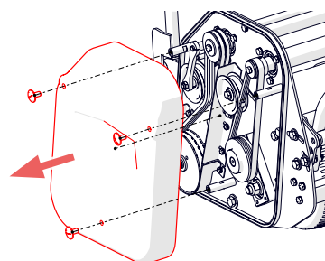
Rys. 16B — Odkręcenie 3 zewnętrznych śrub i zdjęcie osłony
