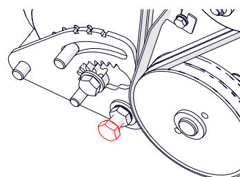
Rys. 27B — Poluzowanie śrub drążka łączącego
