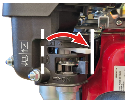
Rys. 12H — Ustawienie dźwigni dławika w położeniu otwartym
