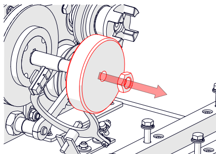
Rys. 17F — Demontaż tarczy hamulcowej
