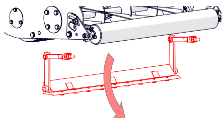
Rys. 18F — Odkręcenie śrub sześciokątnych ostrza tnącego po prawej stronie
