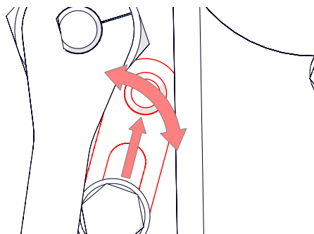
Rys. 24A — Obrócenie i przesunięcie prowadnicy do skrajnego położenia
