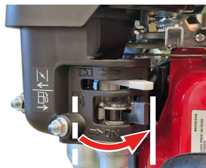
Rys. 12C — Dźwignia paliwa w położeniu otwartym
