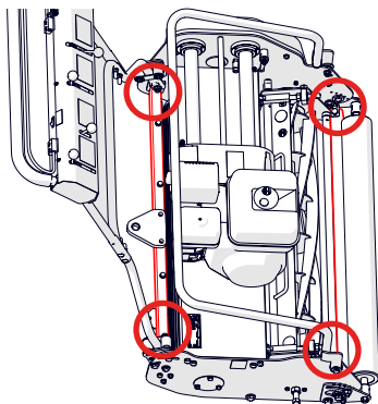
Fig.25. Punkty mocowania do transportu.
