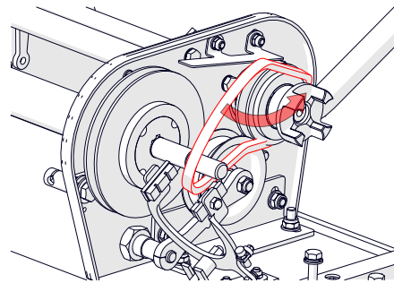
Rys. 17G — Wymiana paska napędowego
