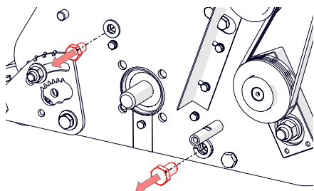
Rys. 18E — Odkręcenie śrub sześciokątnych ostrza tnącego po lewej stronie
