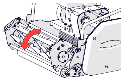
Rys. 7D — Wyjęcie kasety
