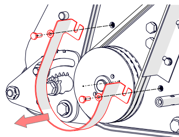
Rys. 16C — Zdjęcie prowadnicy paska
