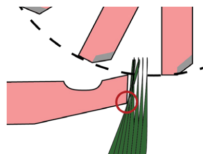
Płaski kąt przedni
