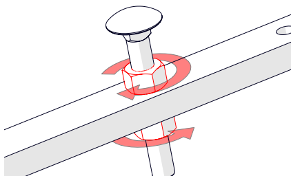
Rys. 8B — Wyregulowanie śruby do żądanej wysokości koszenia i dokręcenie nakrętki (w powyższym przykładzie ustawiono wysokość na 25 mm)
