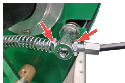
Rys. 17J — Napinanie poprzez odpowiednią regulację nakrętek
