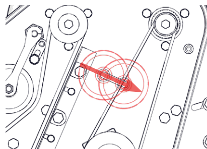
Rys. 16J — Wyregulowanie koła pasowego, by zwiększyć napięcie paska
