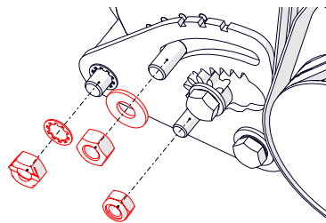
Rys. 27A — Odkręcenie trzech śrub w przedstawiony sposób
