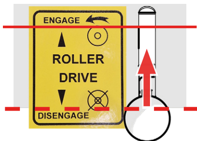
Rys. 14B — Załączanie dźwigni zmiany biegów
