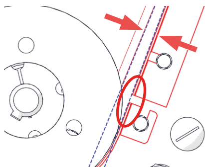
Rys. 16E — Należy upewnić się, że obie prowadnice paska są wypoziomowane (tj. nie ma stopnia) (oznaczone kołem) oraz że między paskiem a prowadnicą paska zachowana jest odpowiednia szczelina (linie)
