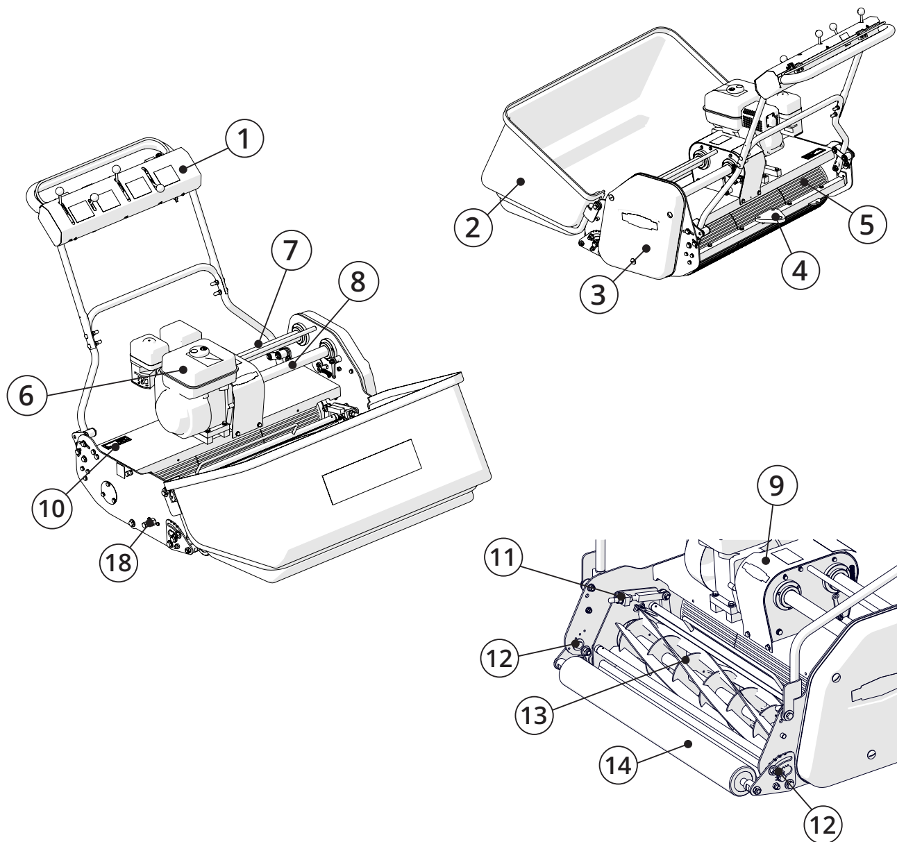
Fig.3. Przegląd elementów maszyny.
