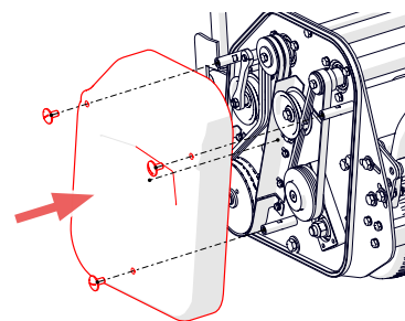
Rys. 16L — Ponowne zakładanie osłony
