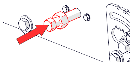
Rys. 7F — Dokręcenie śruby mocującej
