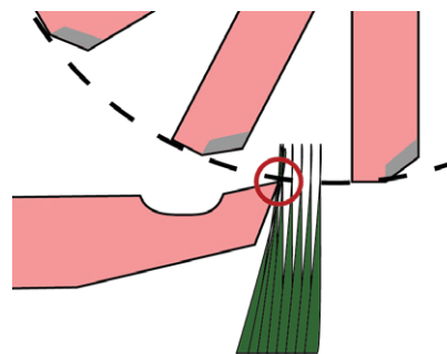
Ujemny kąt przedni
