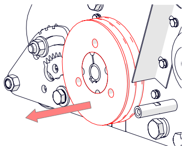
Rys. 18D — Zdjęcie koła pasowego
