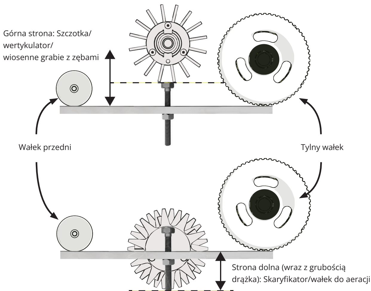
Fig.9. Pomiar drążka regulacyjnego dla kaset pracujących powyżej/poniżej gruntu
