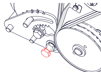
Fig. 25B - Loosen the tie-bar bolt.
