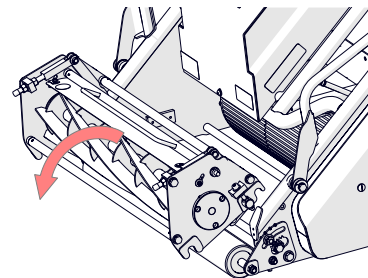
Fig. 8E - Lift the cassette out
