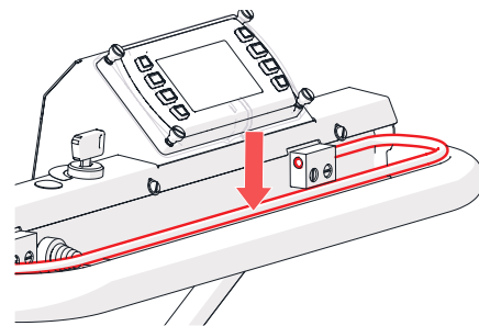
Fig. 15B - Depress the OPC
