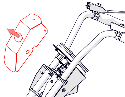
Fig.12C - Remove top console.
