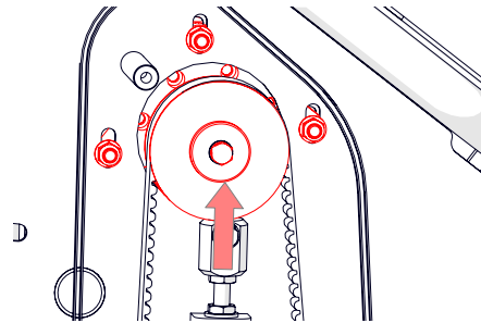
Fig. 19F - Replace the belt.
